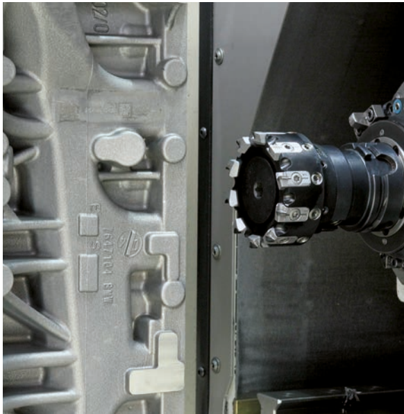
Abbildung 14: Referenzprozess R6
