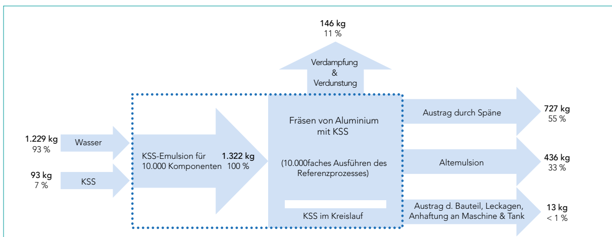
Abbildung 19: Beispielhafte Darstellung einer KSS-Massenbilanz für den Referenzprozess R6 mit KSS
