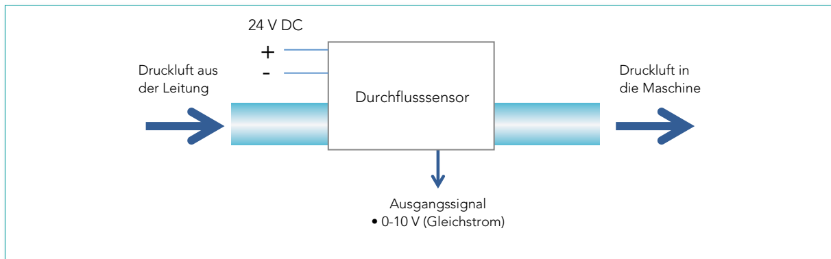
Abbildung 17: Messung des Druckluftverbrauchs
