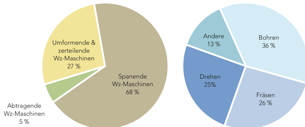
Abbildung 8: Anteile der in Deutschland produzierten Werkzeugmaschinen (links); Zeitanteile der verschiedenen spanenden Bearbeitungsverfahren aus Anwenderbefragung (rechts) 14
