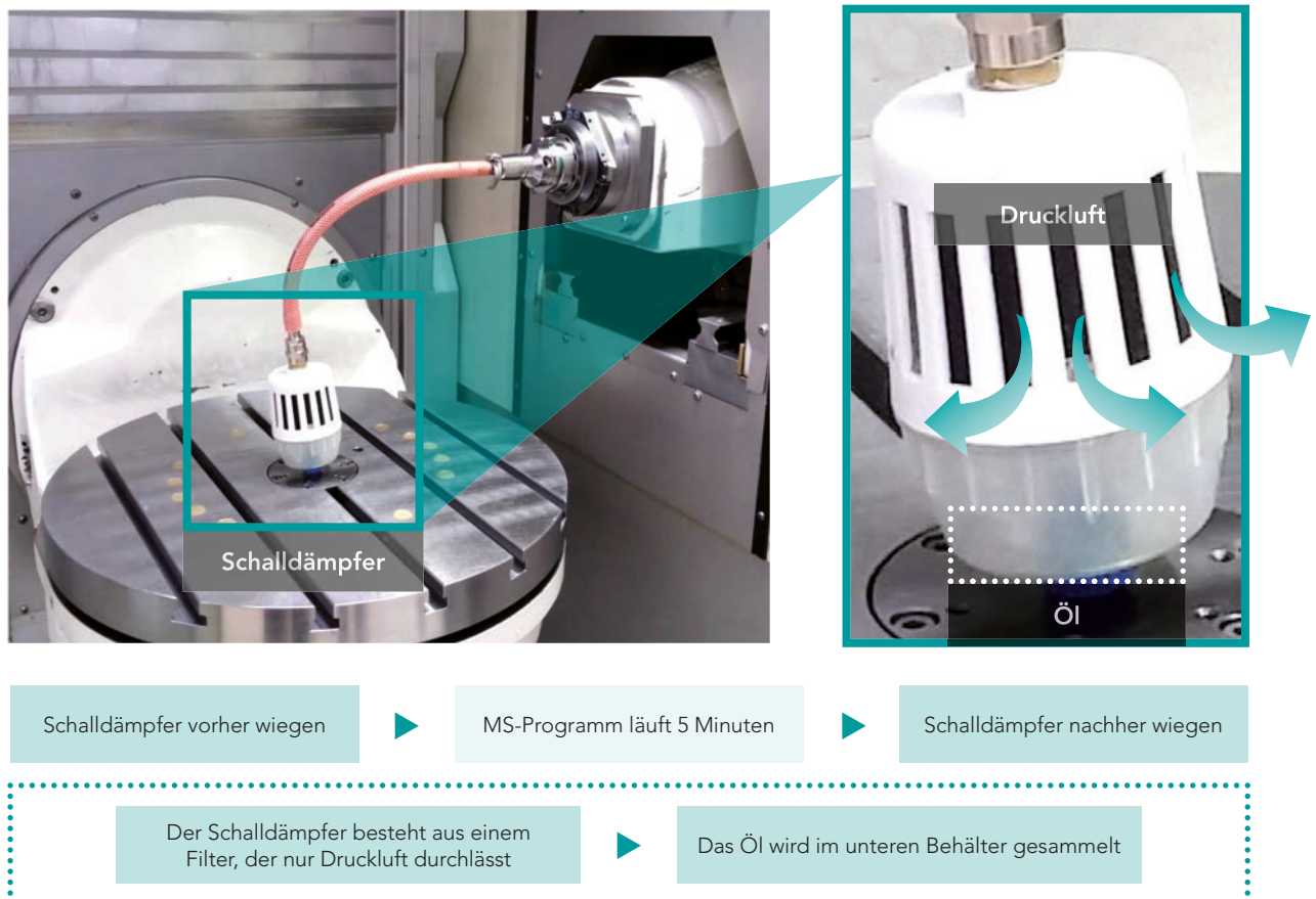
Abbildung 21: Vorgehensweise zur Ermittlung des MMS-Verbrauchs
