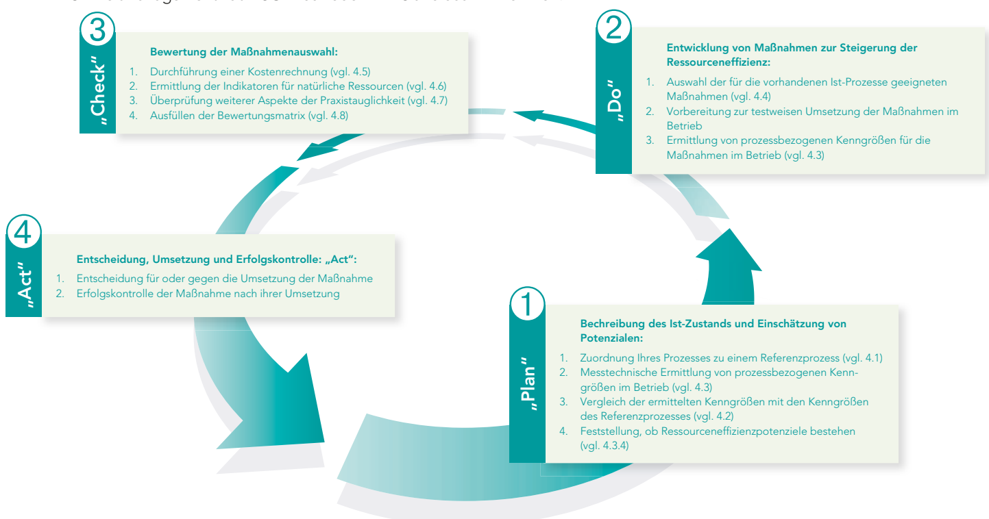
Abbildung 12: Vorgehensweise zur Ausschöpfung von Ressourceneffizienzpotenzialen (PDCA-Zyklus) für die spanende Bearbeitung
