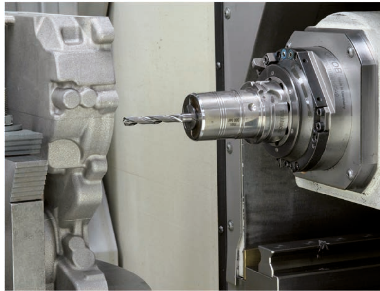
Abbildung 15: Referenzprozess R1
