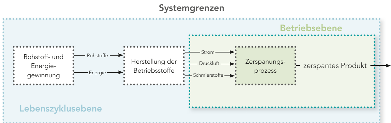
Abbildung 22: Angepasste Systemgrenze mit den relevanten prozessbezogenen Kenngrößen
