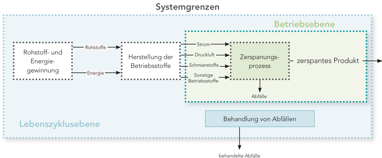
Abbildung 6: Systemgrenzen für die Betrachtungsräume „Betriebsebene“ und „Lebenszyklusebene“
